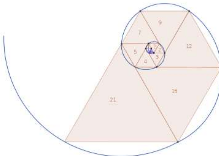
Figura 2 – Espiral de Padovan
