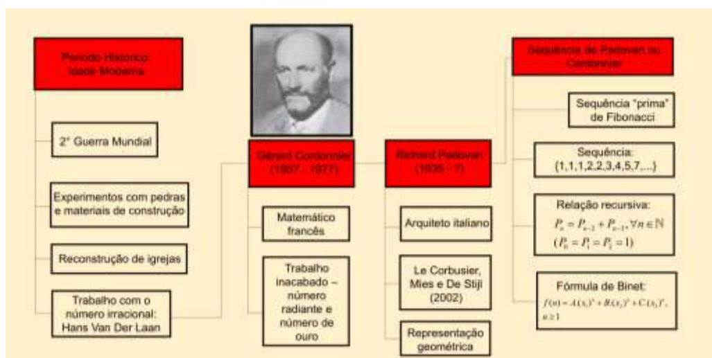
Figura 3 – Campo Epistêmico-Matemático
