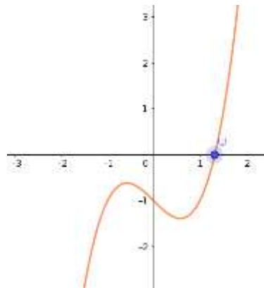
Figura 4 – Gráfico da equação característica de Padovan
